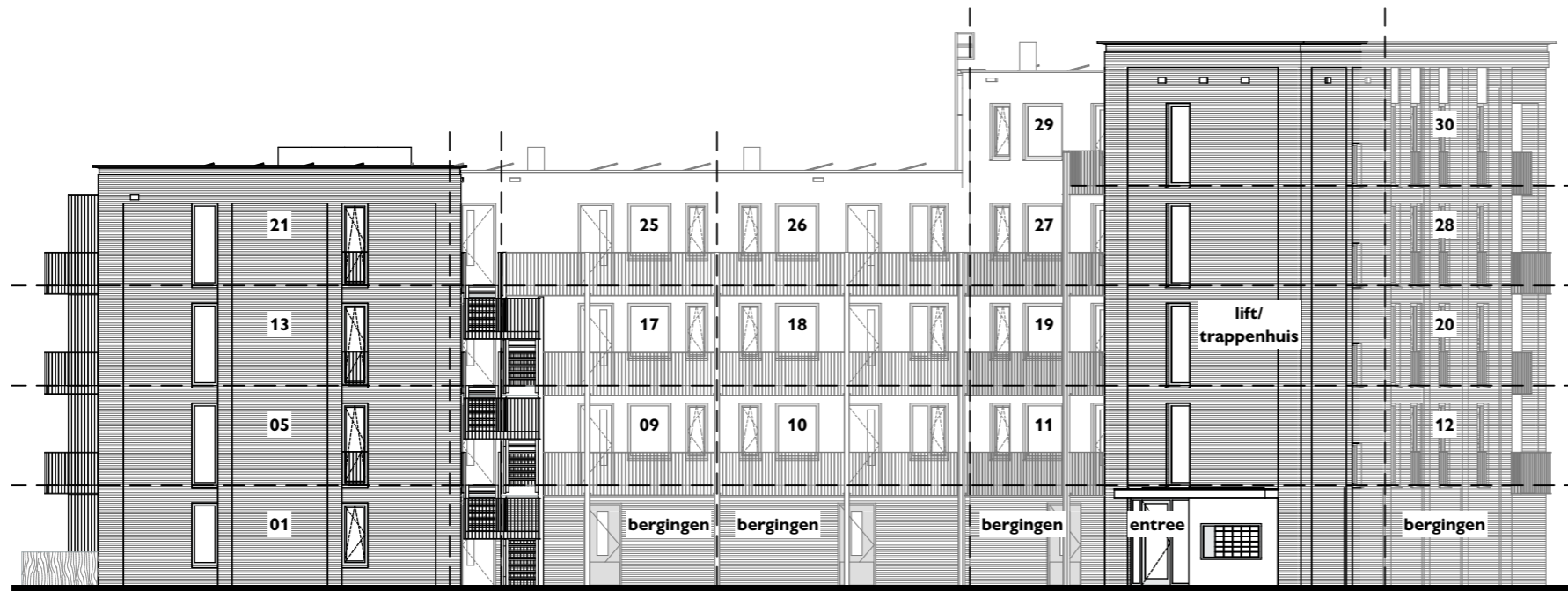
Oostgevel
