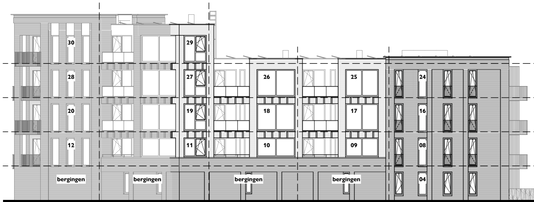
Westgevel rechts
