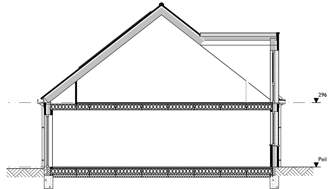
Doorsnede B-B
