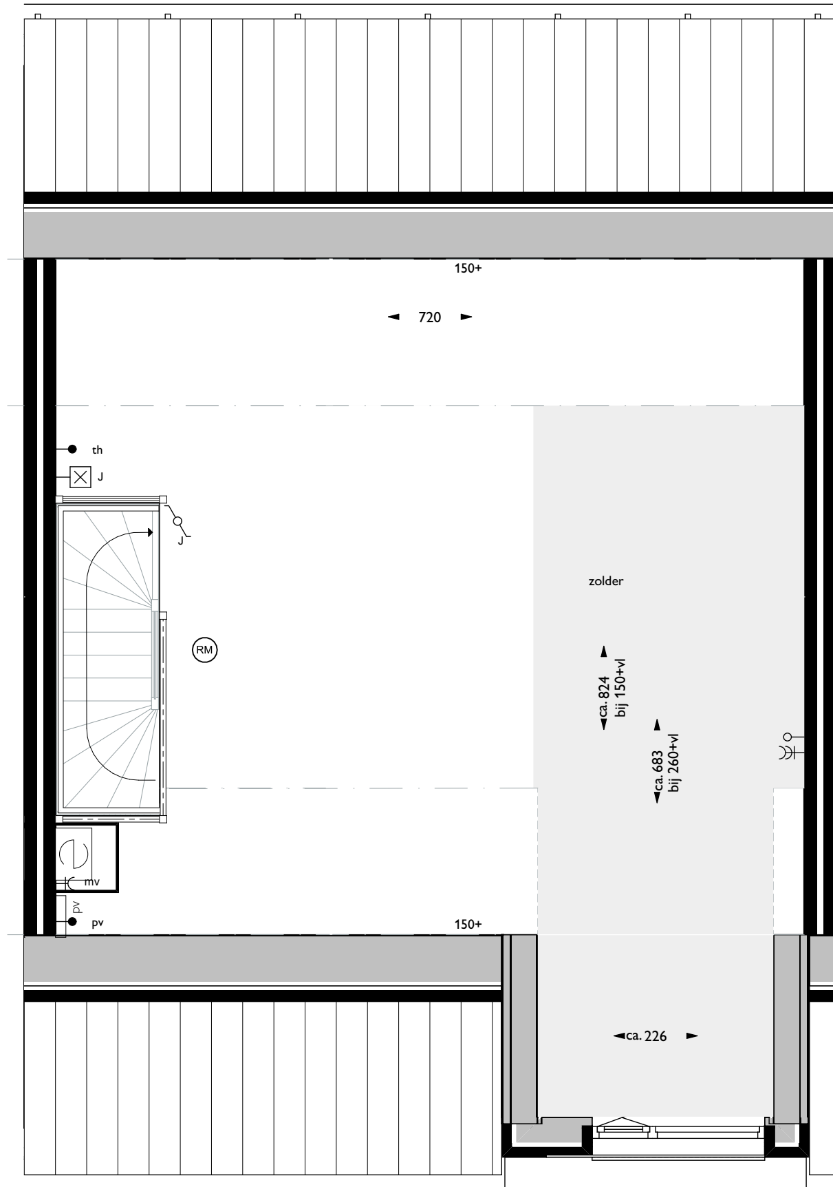
bouwnummer 67 verdieping
