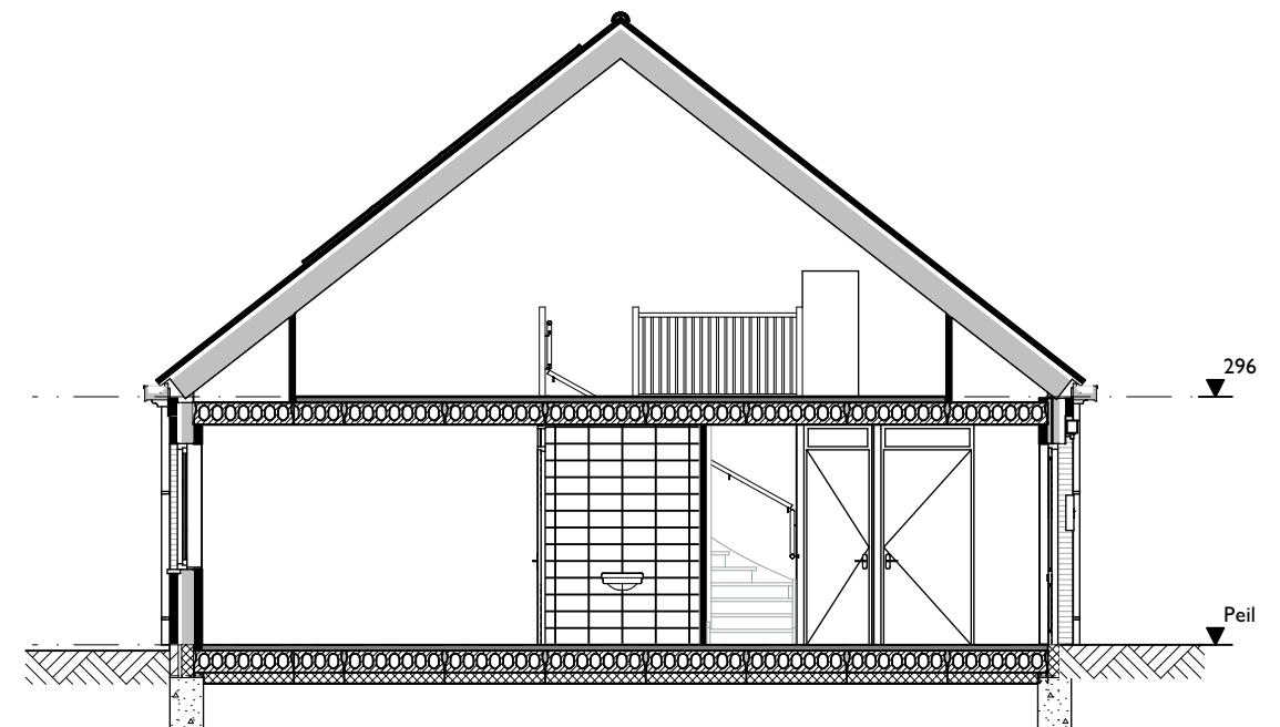
Doorsnede A-A
