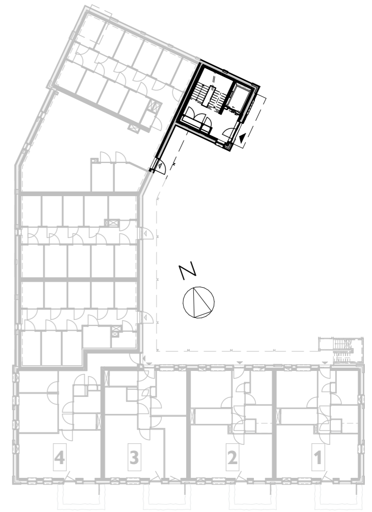
Begane grond
