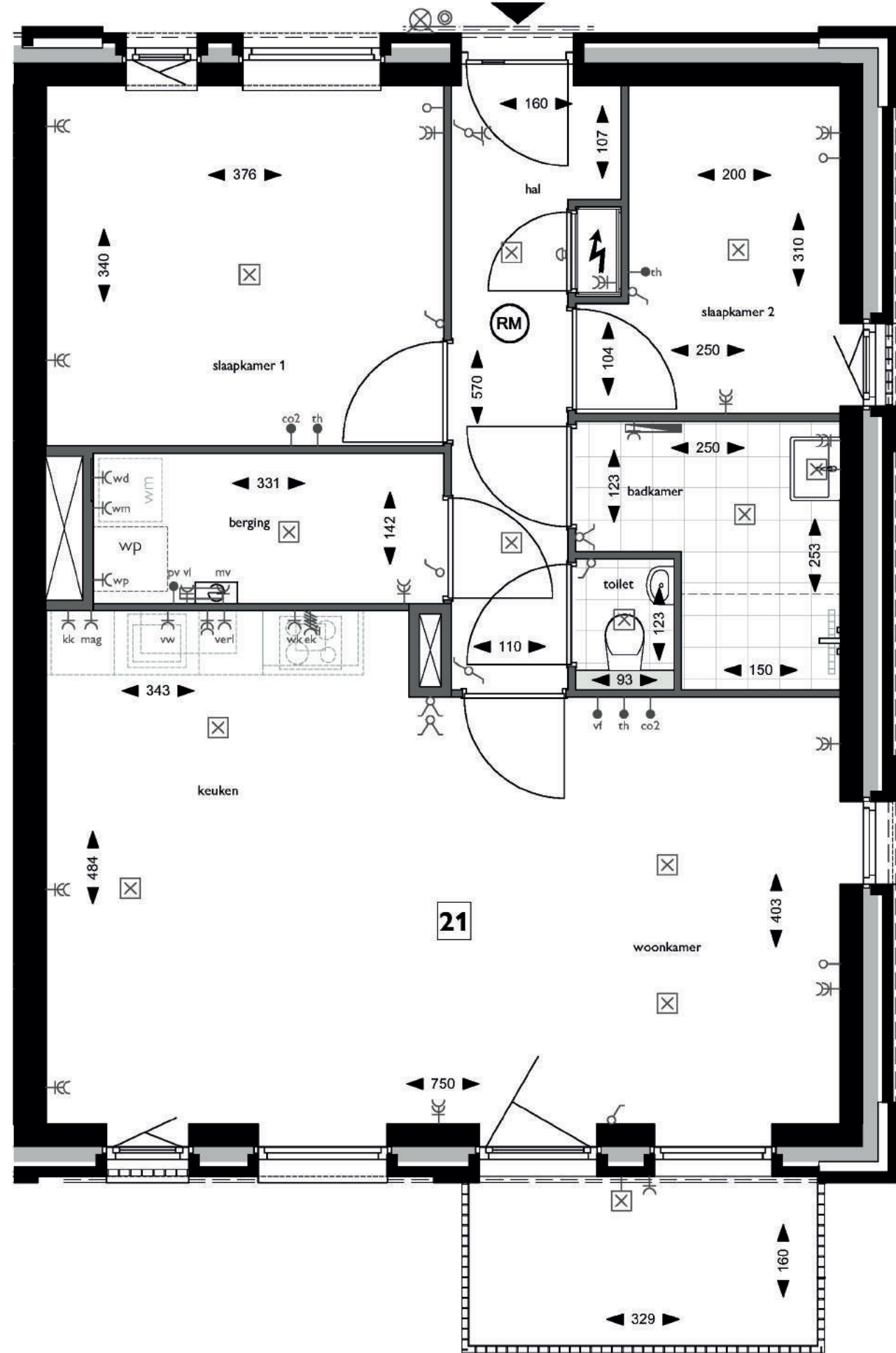
Plattegrond, Blok A - 3e verdieping - appartement 21
