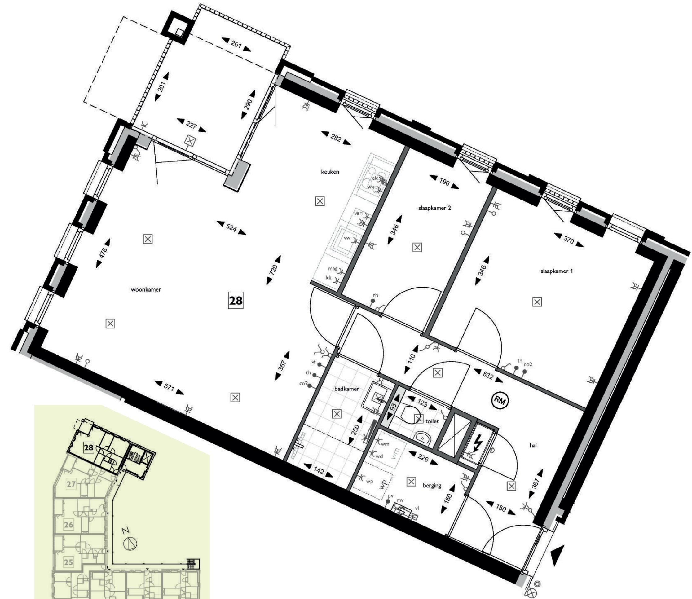
Plattegrond, Blok A - 3e verdieping - appartement 28
