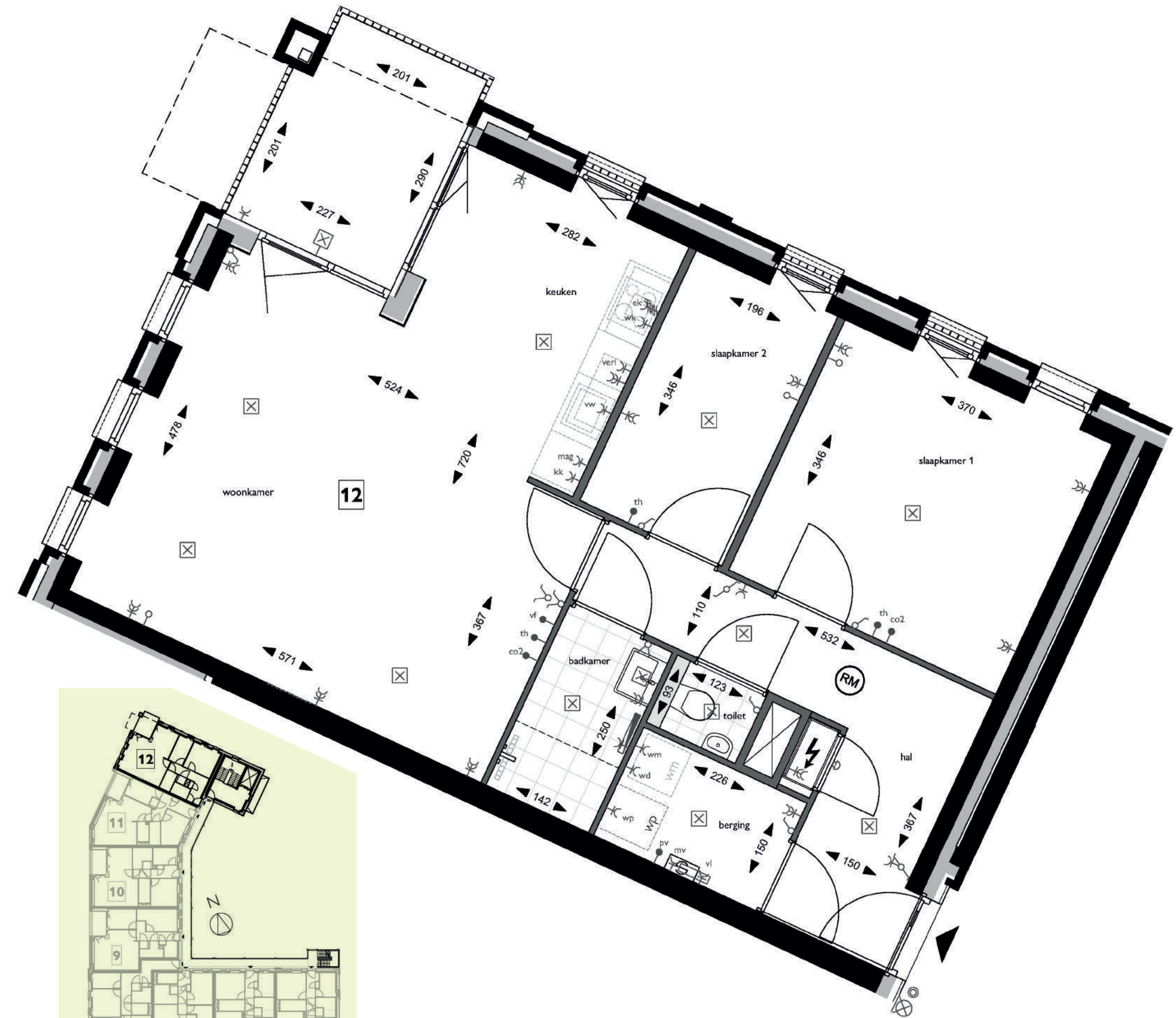
Plattegrond, Blok A - 1e verdieping - appartement 12
