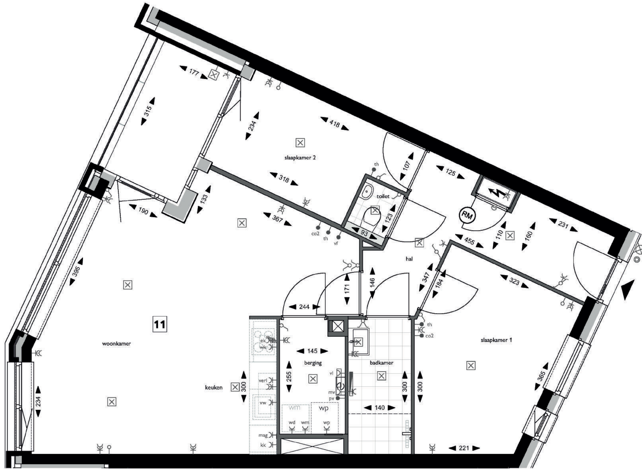
Plattegrond, Blok A - 1e verdieping - appartement 11
