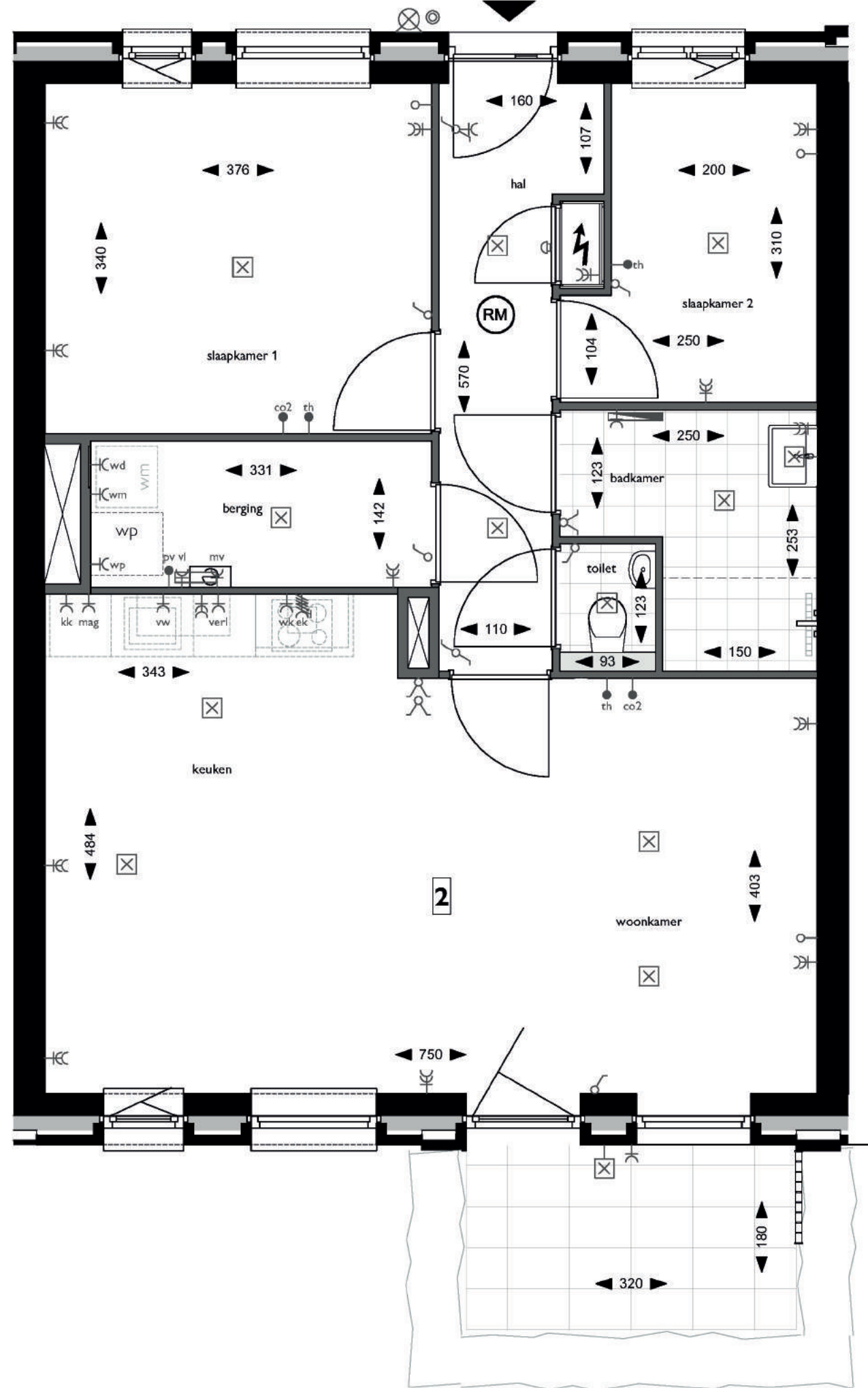
Plattegrond, Blok A - begane grond - appartement 2
