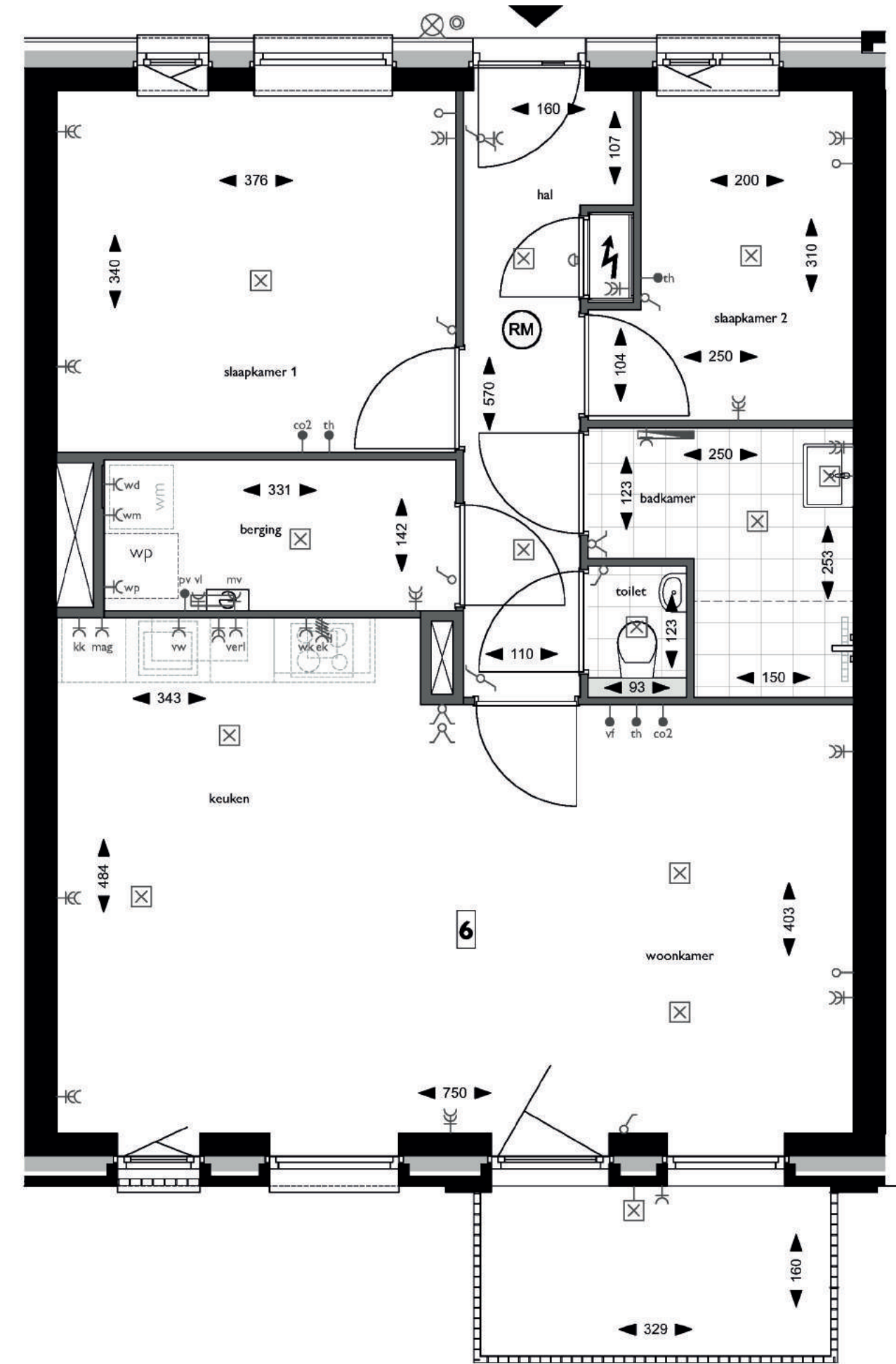
Plattegrond, Blok A - 1e verdieping - appartement 6
