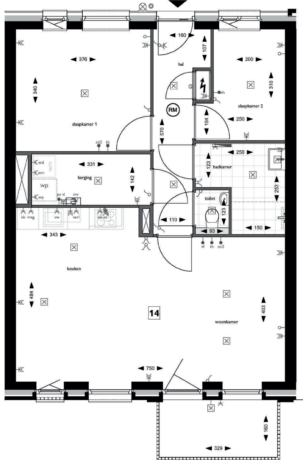
Plattegrond, Blok A - 2e verdieping - appartement 14
