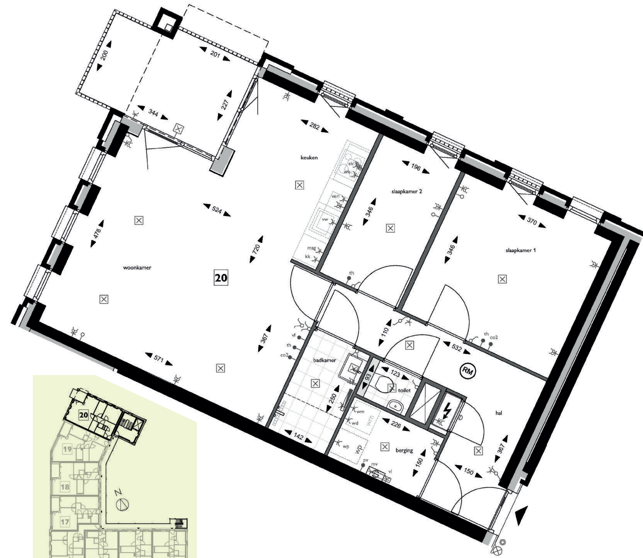
Plattegrond, Blok A - 2e verdieping - appartement 20
