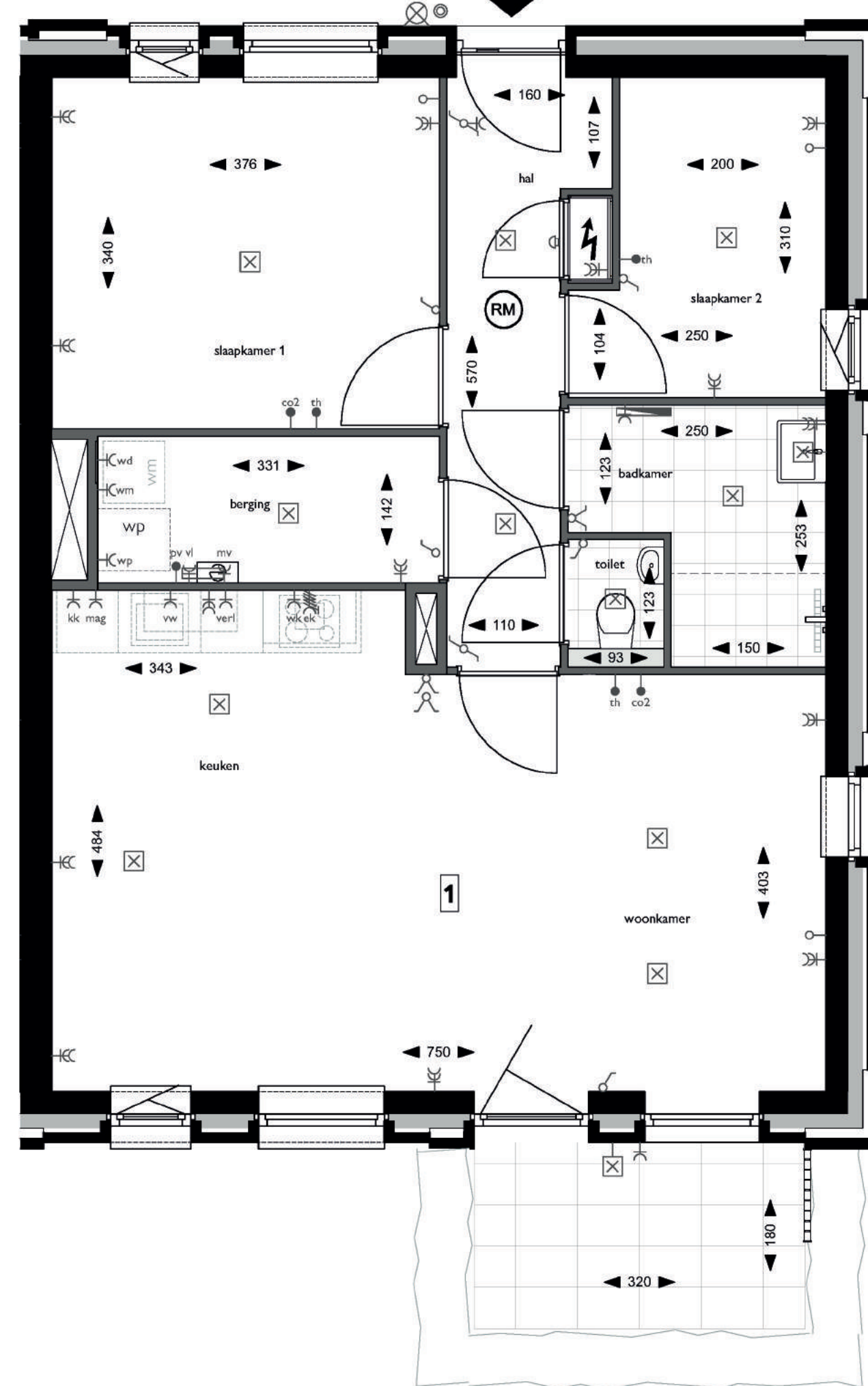
Plattegrond, Blok A - begane grond - appartement 1
