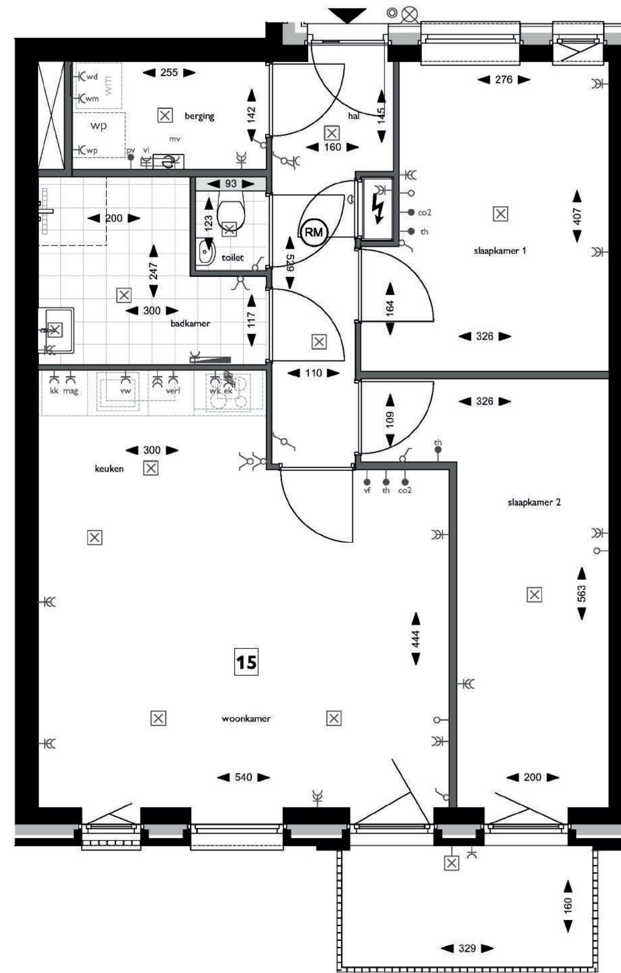
Plattegrond, Blok A - 2e verdieping - appartement 15
