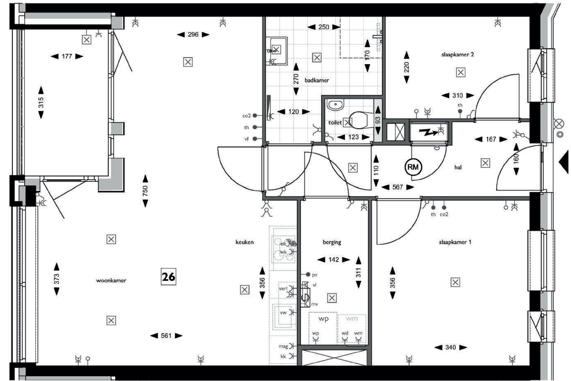
Plattegrond, Blok A - 3e verdieping - appartement 26
