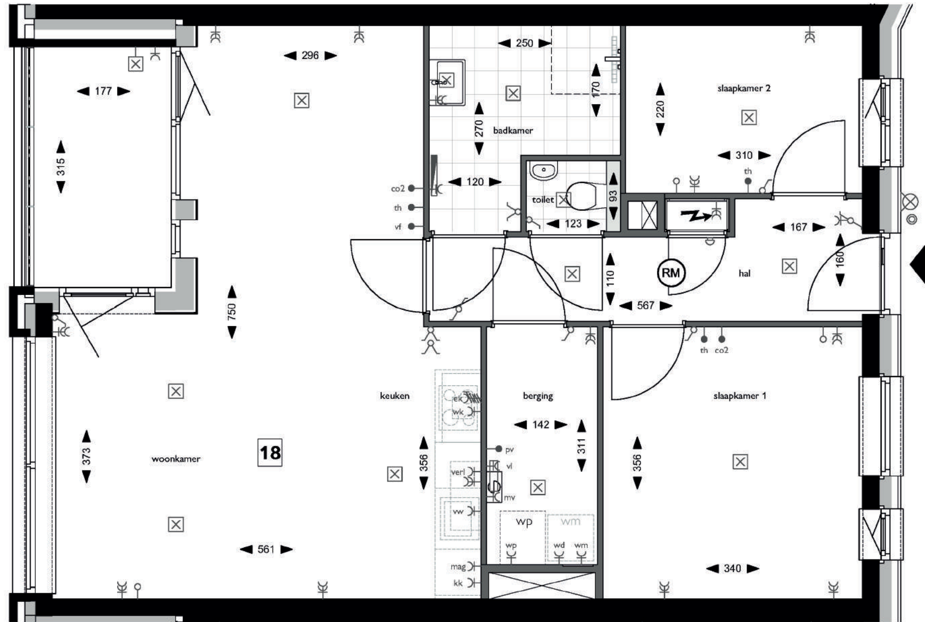
Plattegrond, Blok A - 2e verdieping - appartement 18
