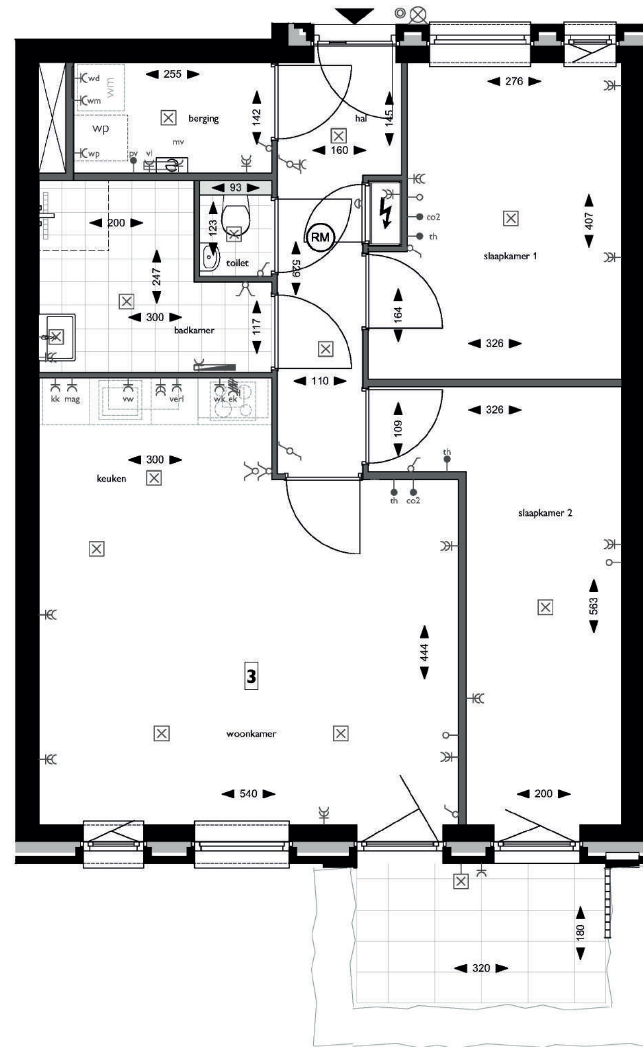
Plattegrond, Blok A - begane grond - appartement 3
