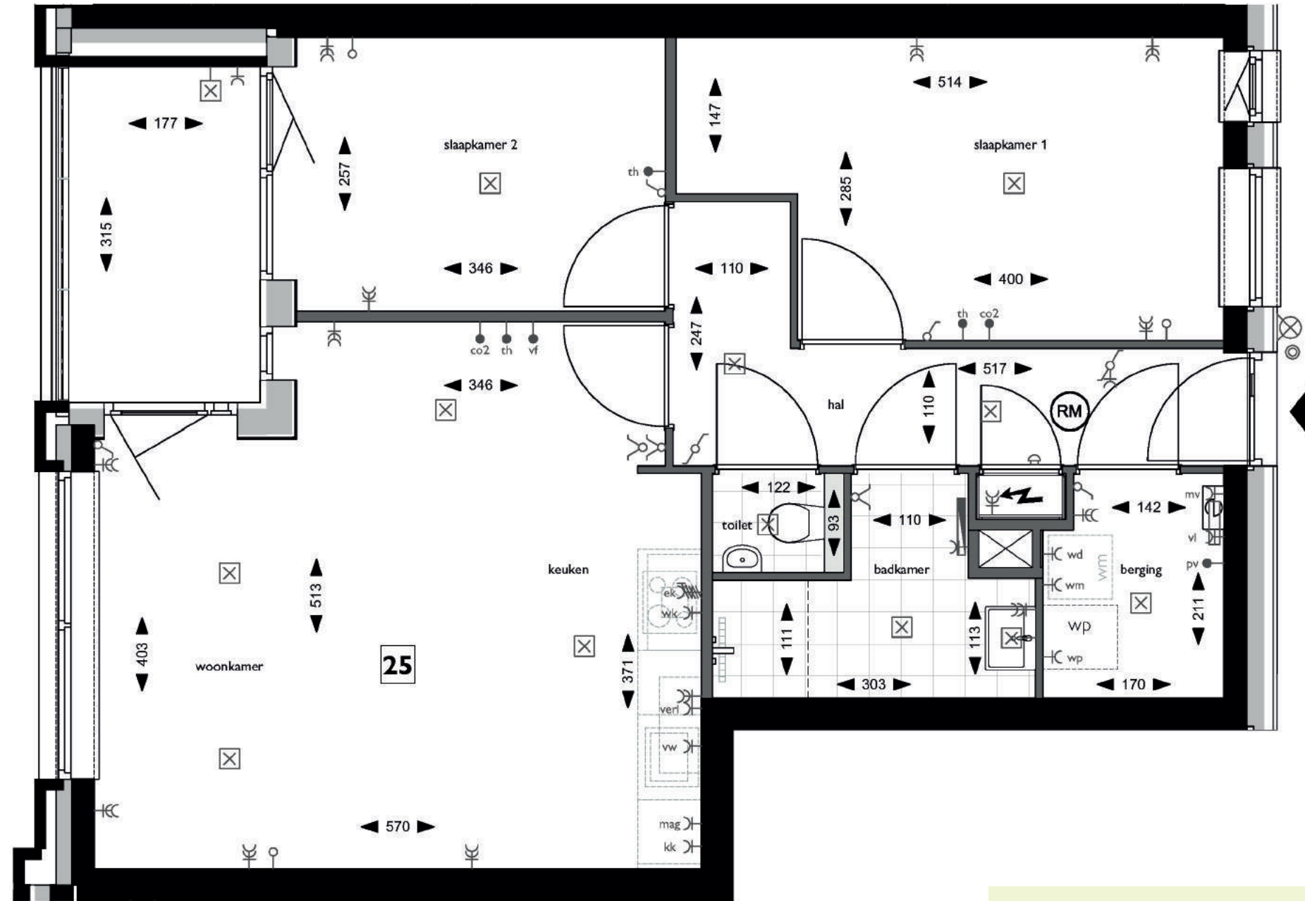
Plattegrond, Blok A - 3e verdieping - appartement 25
