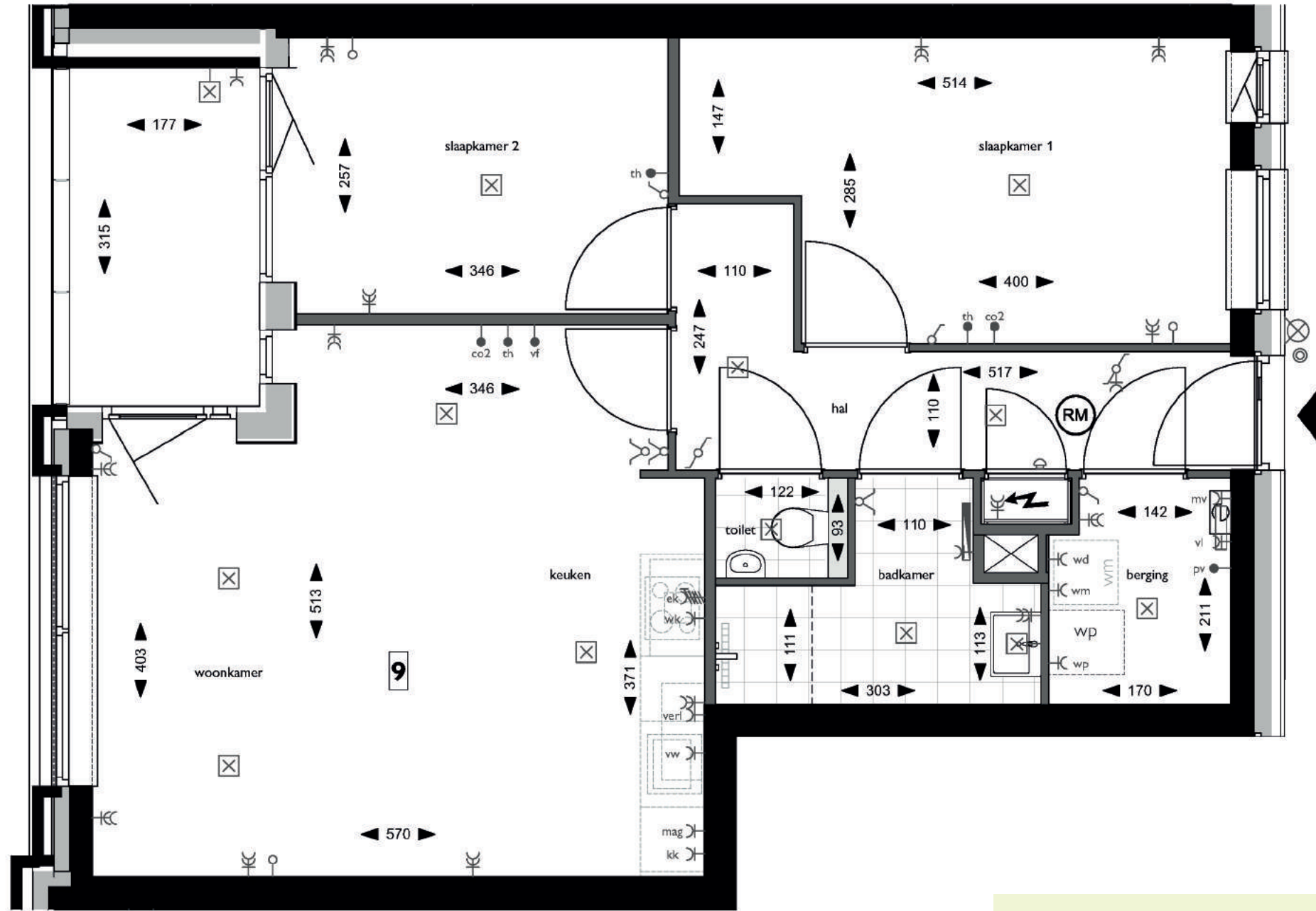
Plattegrond, Blok A - 1e verdieping - appartement 9
