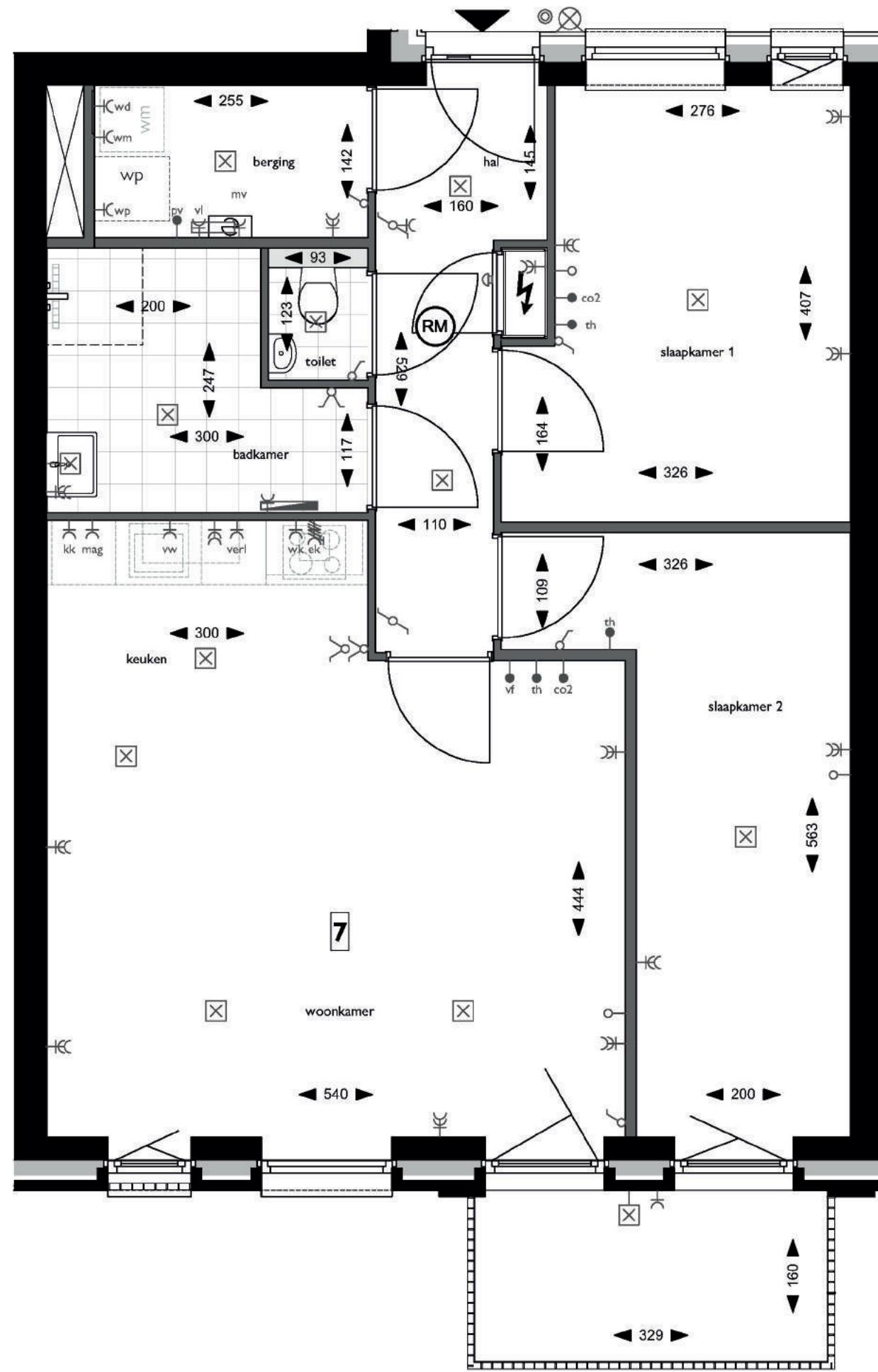
Plattegrond, Blok A - 1e verdieping - appartement 7
