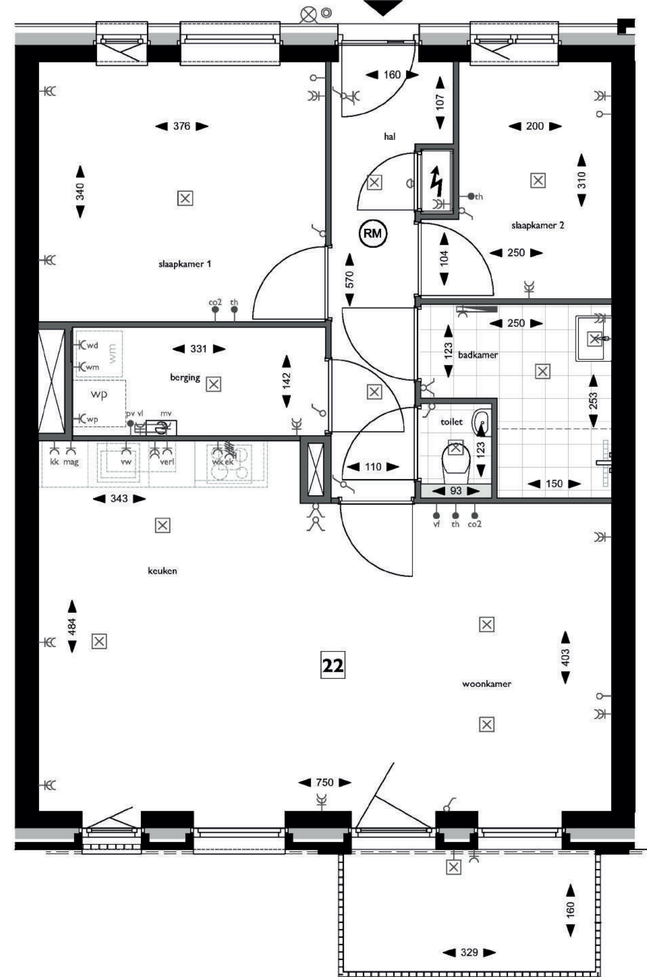
Plattegrond, Blok A - 3e verdieping - appartement 22
