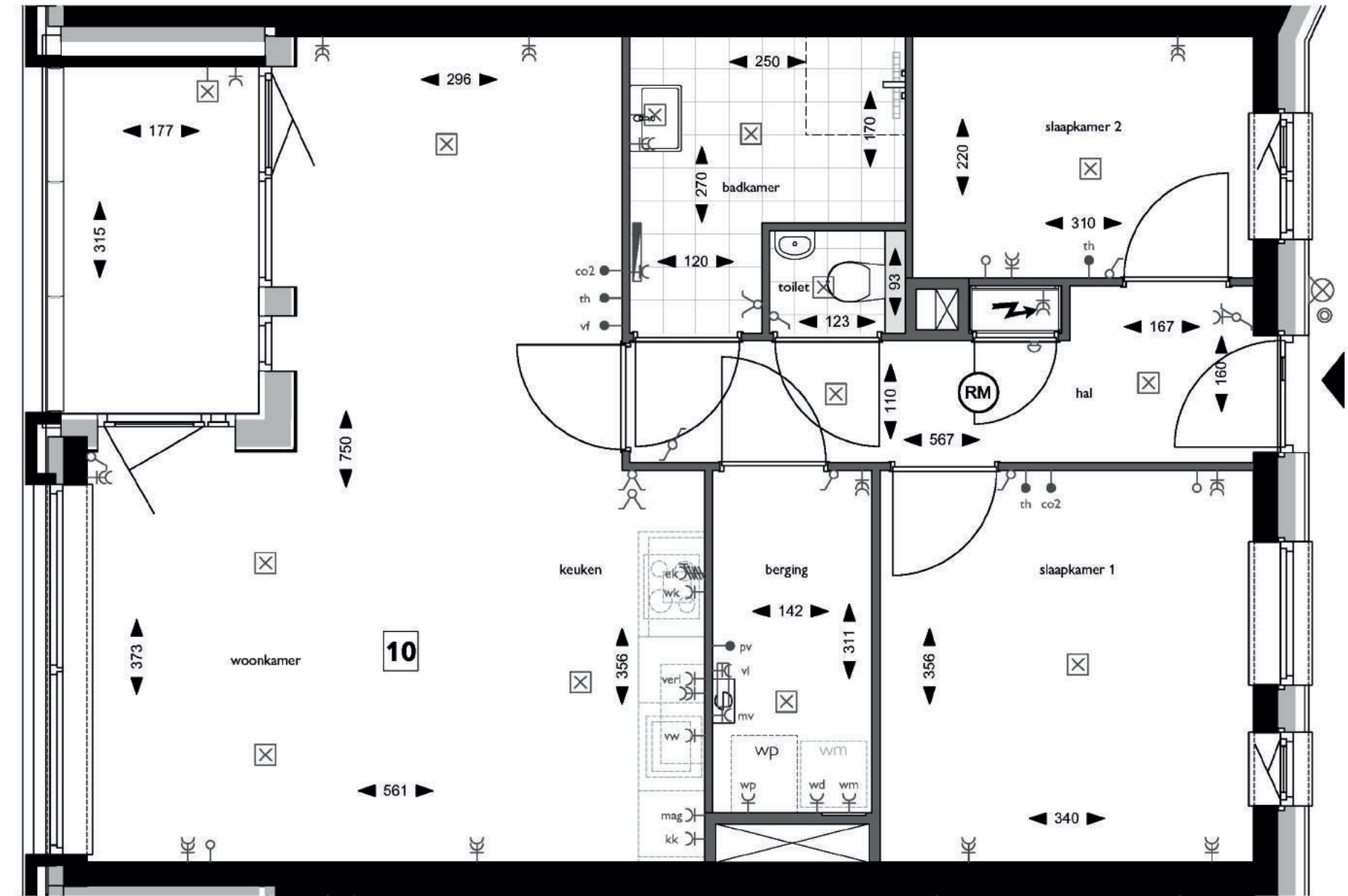
Plattegrond, Blok A - 1e verdieping - appartement 10
