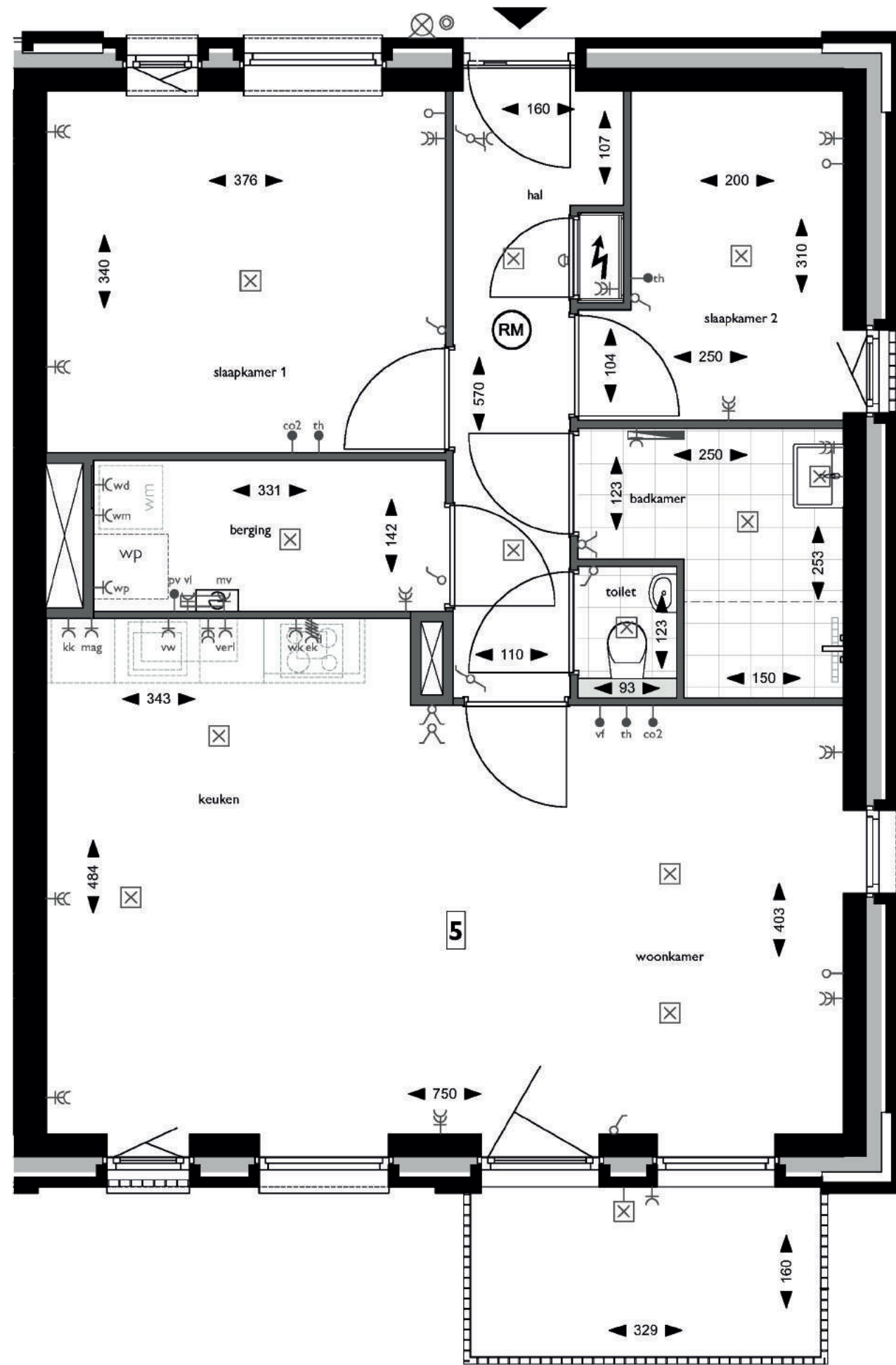
Plattegrond, Blok A - 1e verdieping - appartement 5
