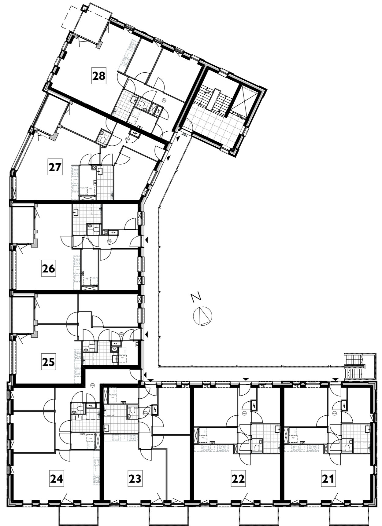
3e verdieping
