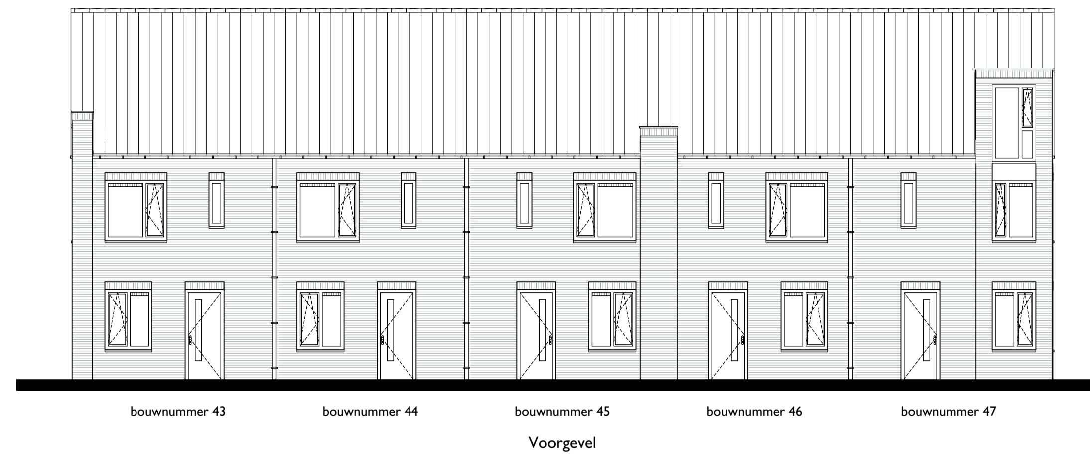
Voorgevel
