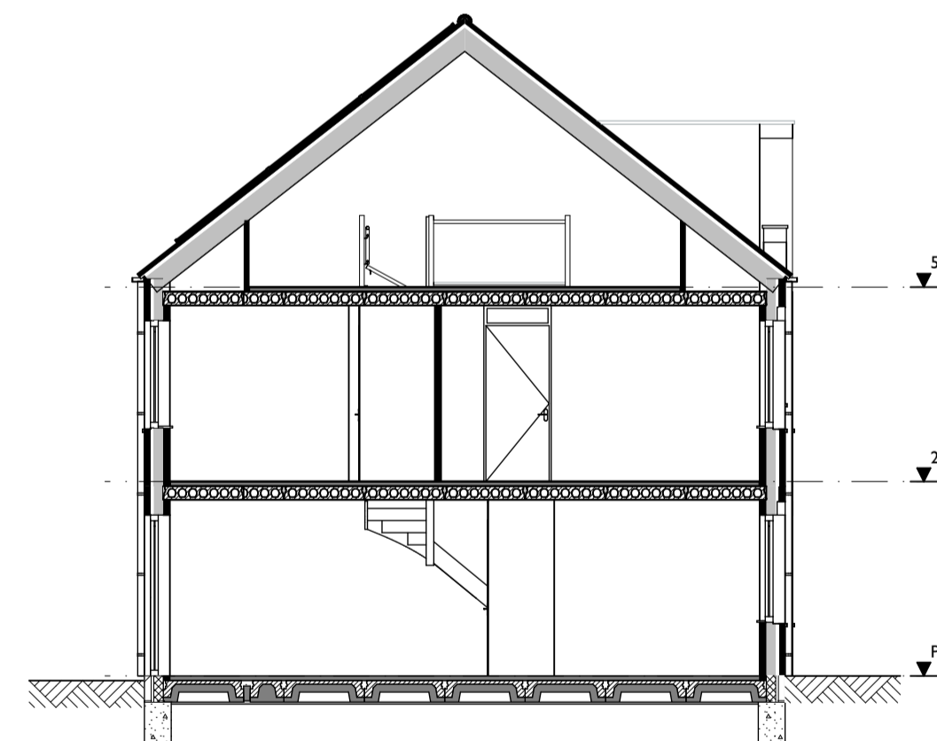
Doorsnede A-A
