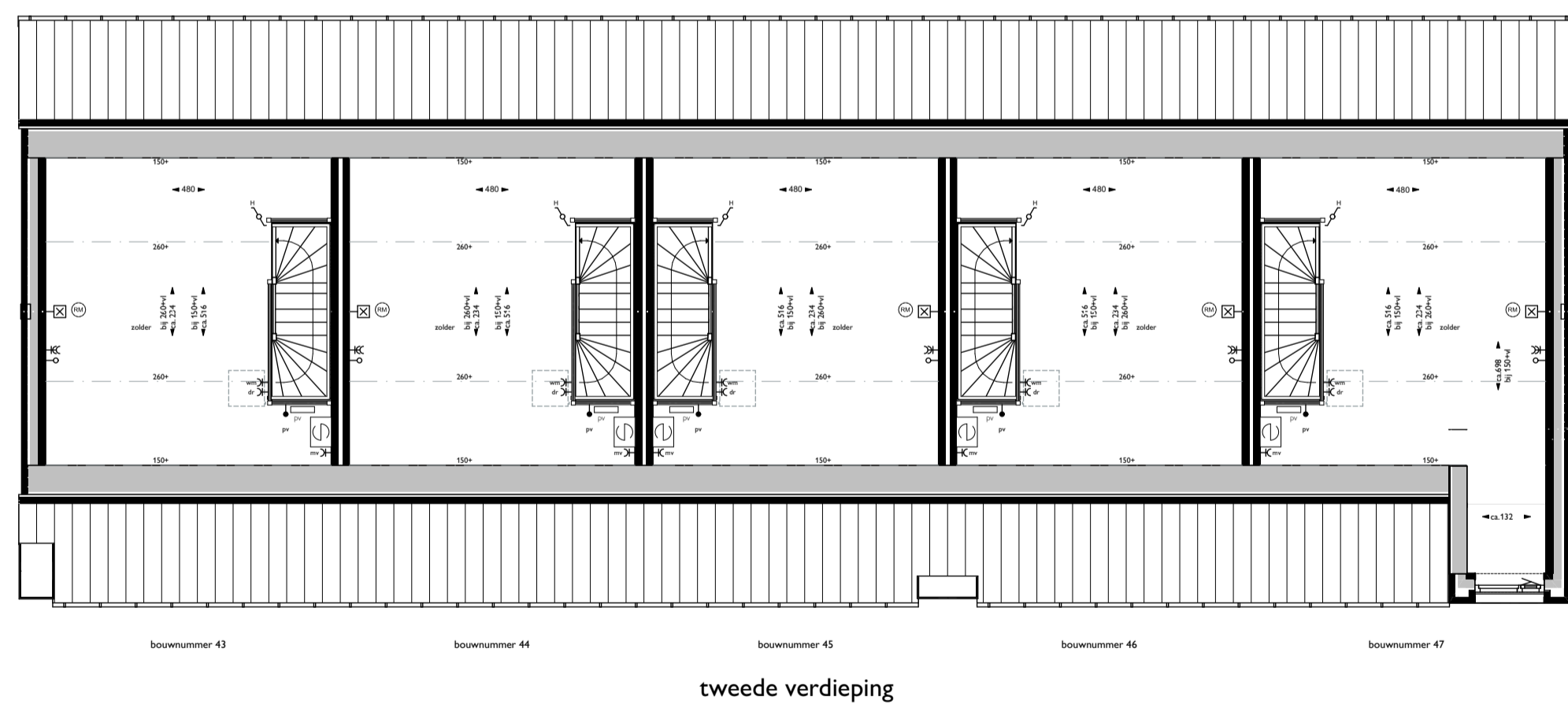
tweede verdieping
