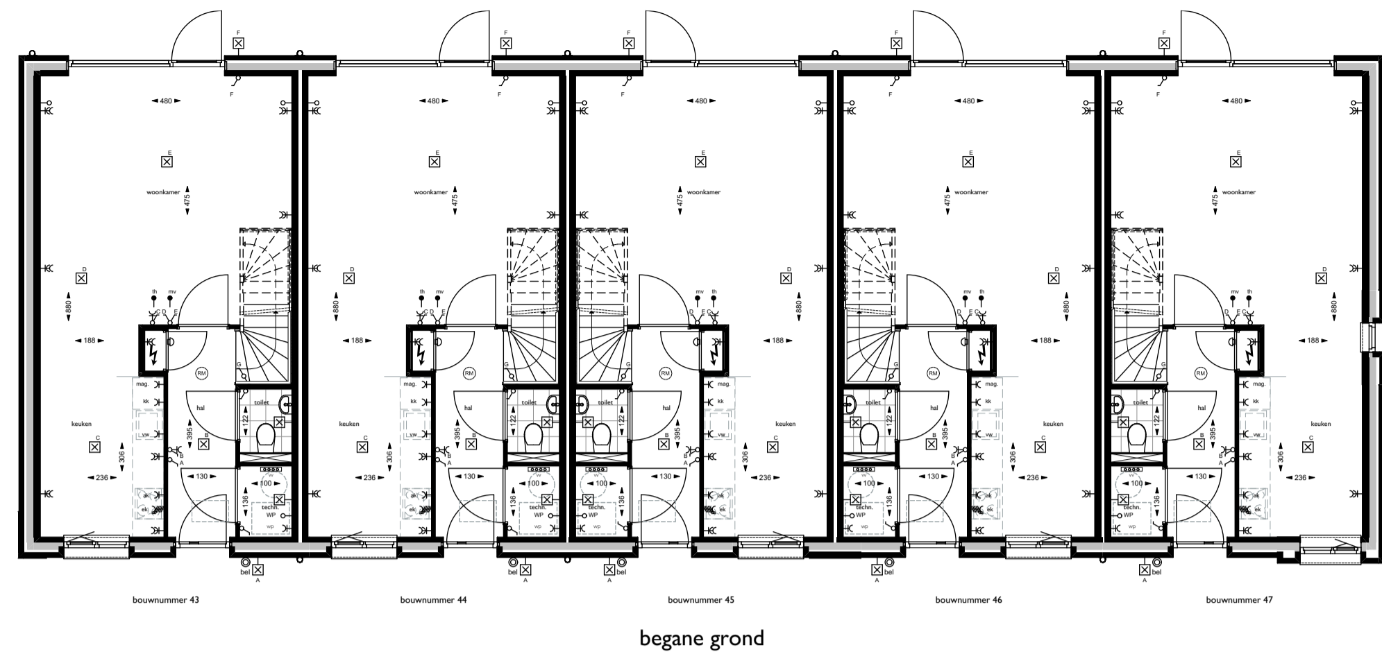
begane grond
