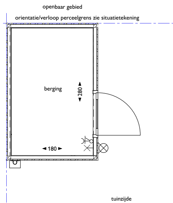
principetekening berging enkel
